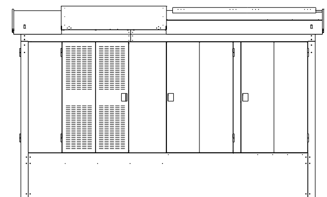
JULKISIVU OIKEALTA
