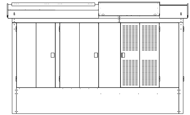
JULKISIVU VASEMMALTA
